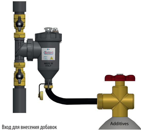
Вход для внесения добавок
