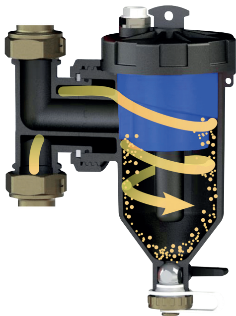
Рис. В1: циклонная фильтрация + отстаивание в шламоотделителе
