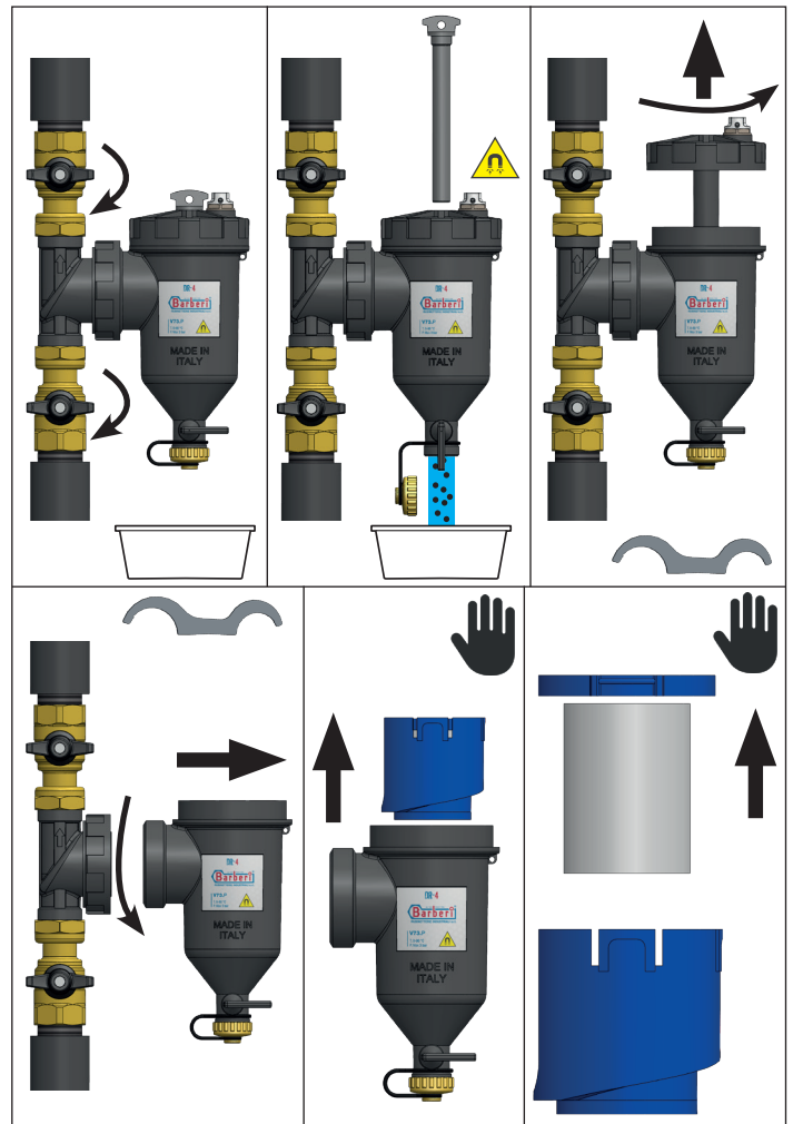
Очистка повышенной интенсивности
