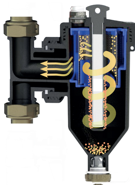
Рис. В3: механическая фильтрация
