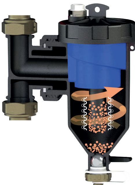
Рис. В2: действие магнита
