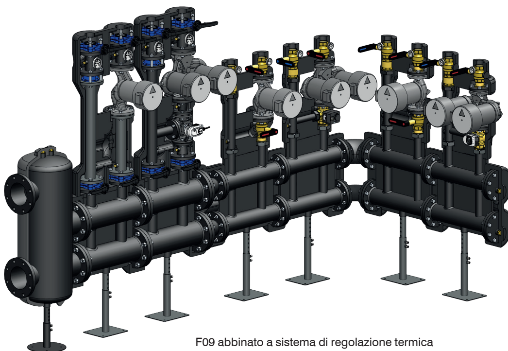
21M.01 abbinato a sistema di regolazione termica realizzato con collettori e gruppi di regolazione da centrale termica
